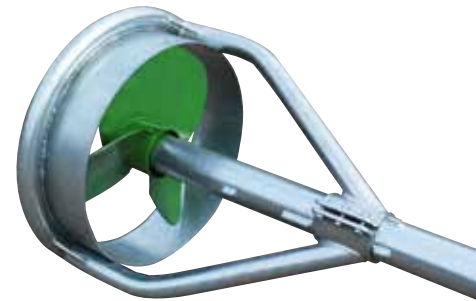
Rührwerkskorb in der Bauart rund
