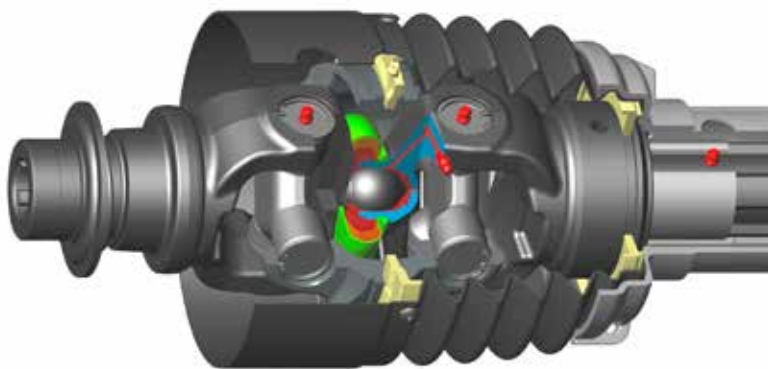
De gepatenteerde 50°-goothoekkoppeling – minder slijtage, ook bij een continue hoek, in vergelijking met een 80°-goothoekkoppeling
